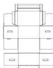
6. กล่อง Tuck Folder
